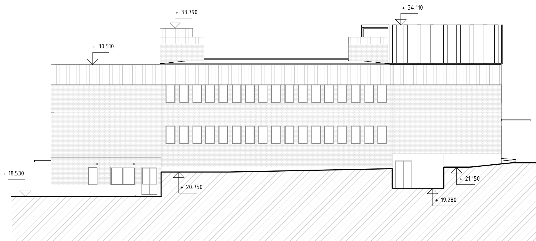
4 - FASAD MOT ÖSTER
