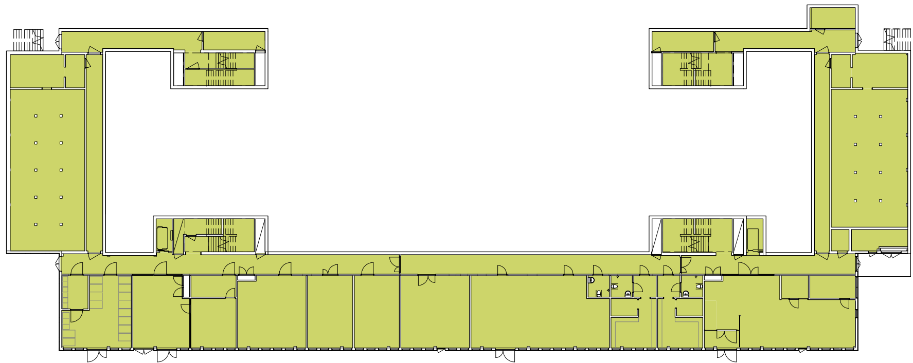
PLAN 09 NTA
