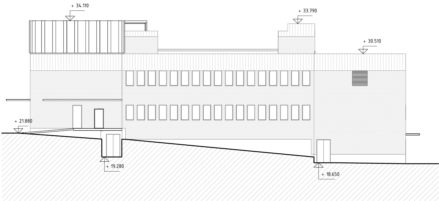
3 - FASAD MOT VÄSTER
