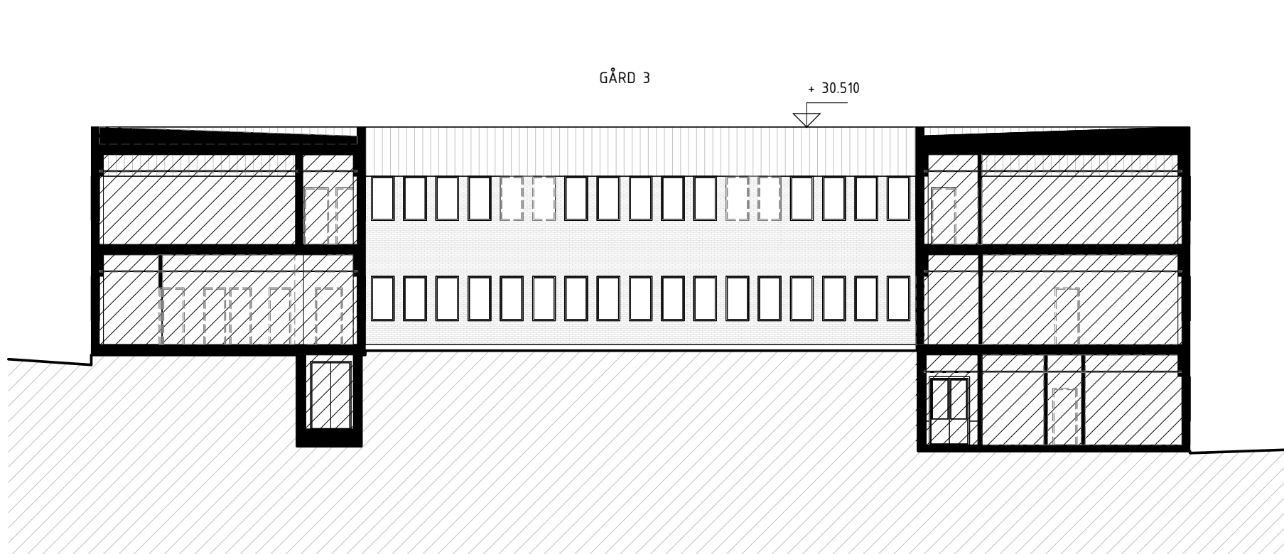
10 - FASAD MOT VÄSTER, GÅRD 3, BEFINTLIG
