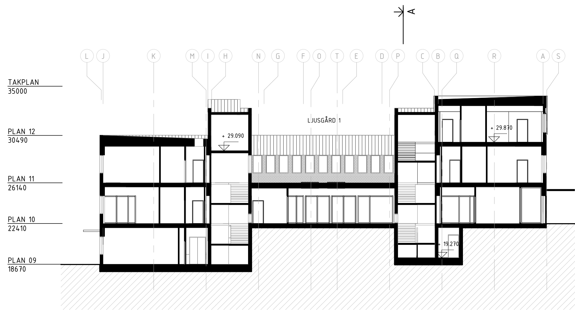
SEKTION B-B
