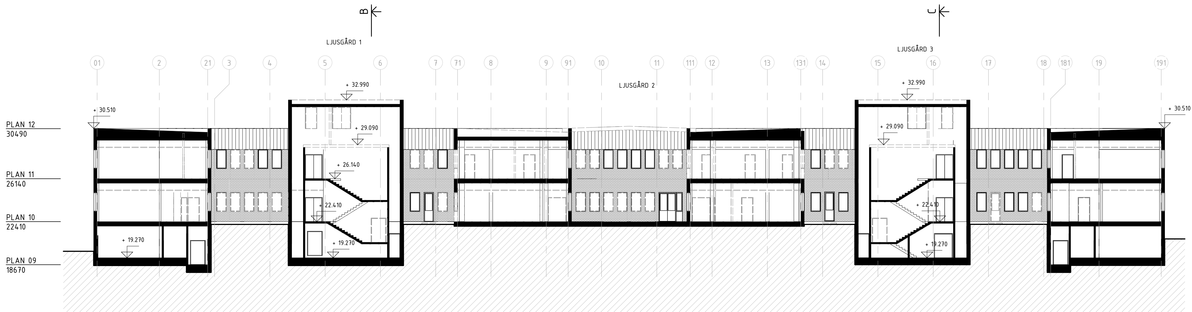
SEKTION A-A, BEFINTLIG
