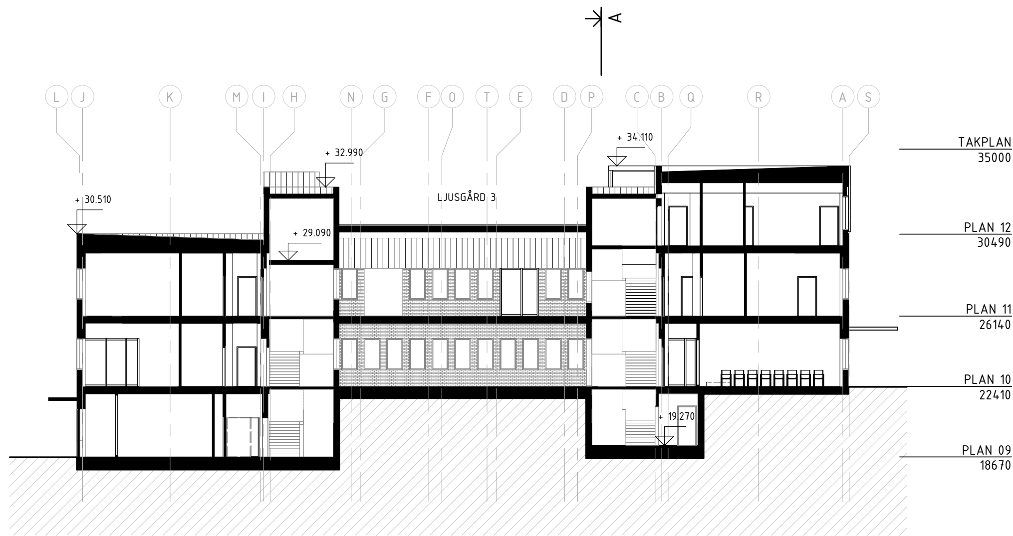
SEKTION C-C
