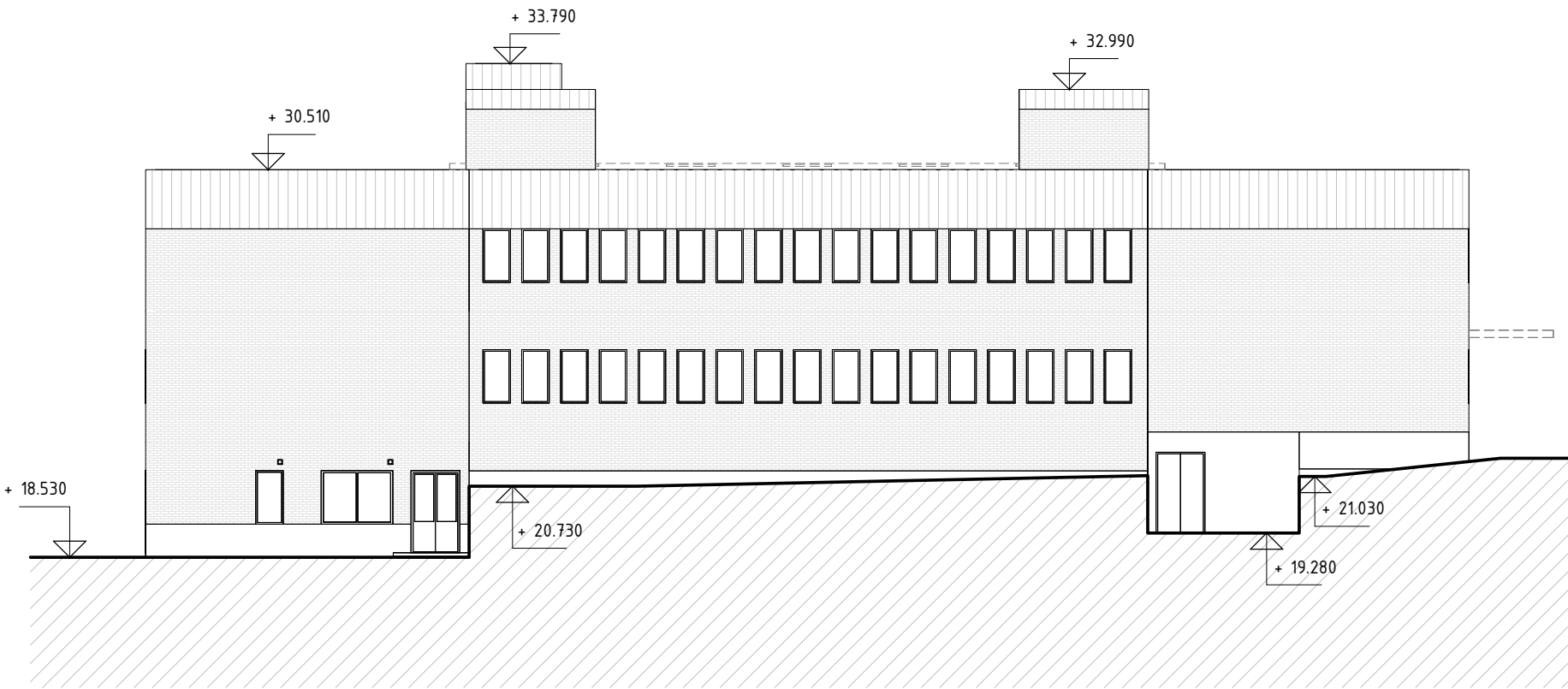
4 - FASAD MOT ÖSTER, BEFINTLIG
