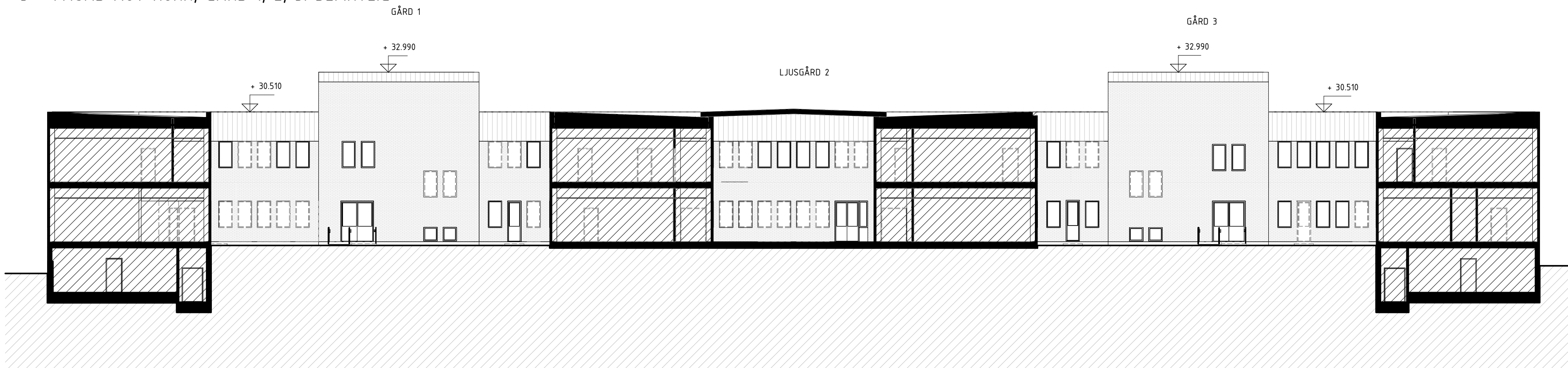
6 - FASAD MOT SÖDER, GÅRD 1, 2, 3. BEFINTLIG
