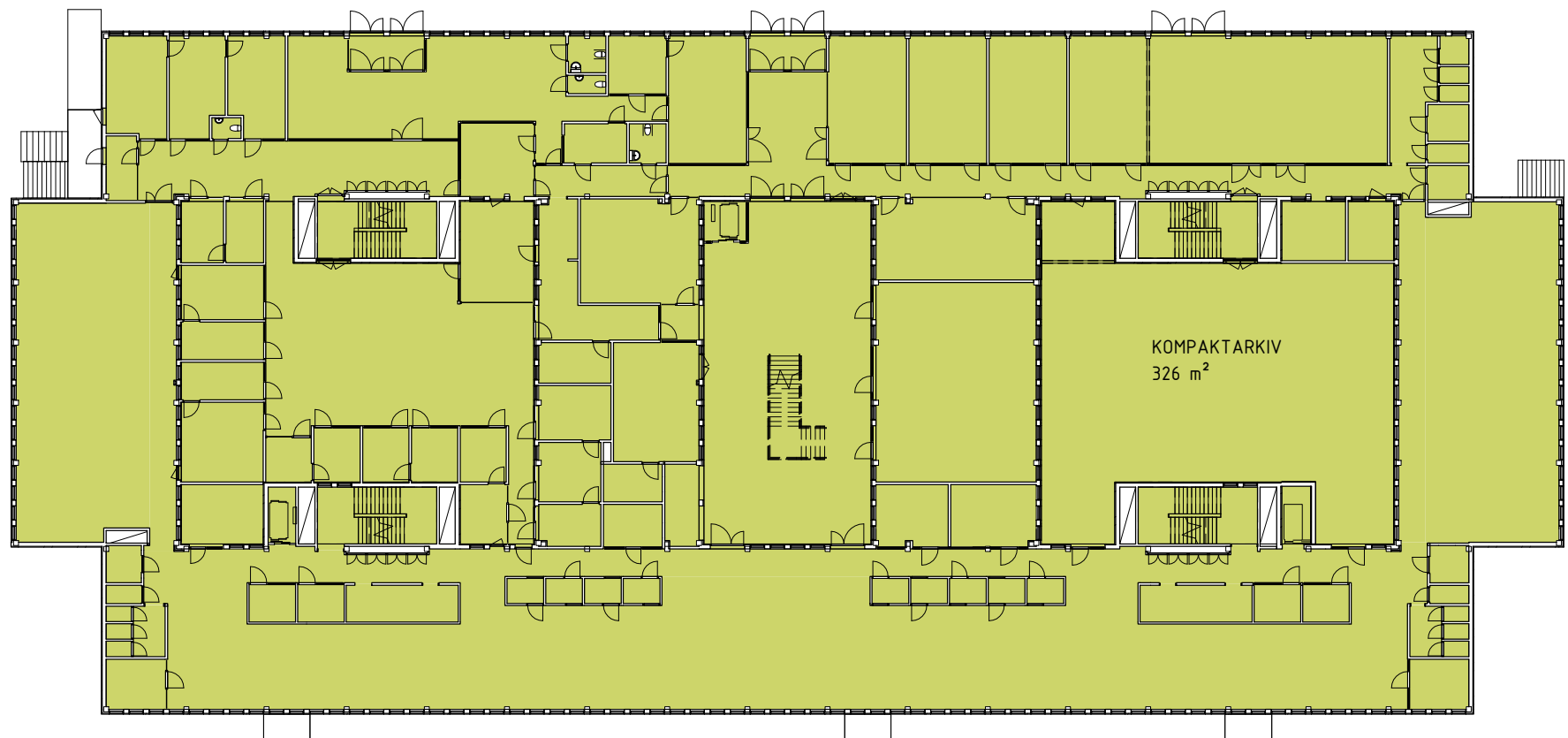
PLAN 10 NTA
