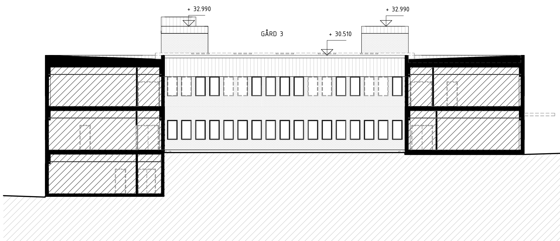
9 - FASAD MOT ÖSTER, GÅRD 3, BEFINTLIG
