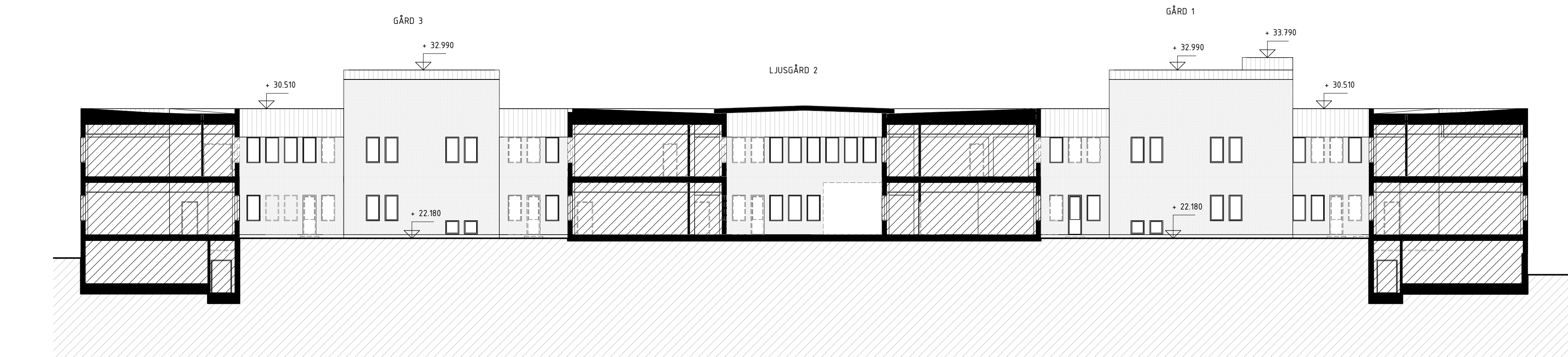
5 - FASAD MOT NORR, GÅRD 1, 2, 3. BEFINTLIG
