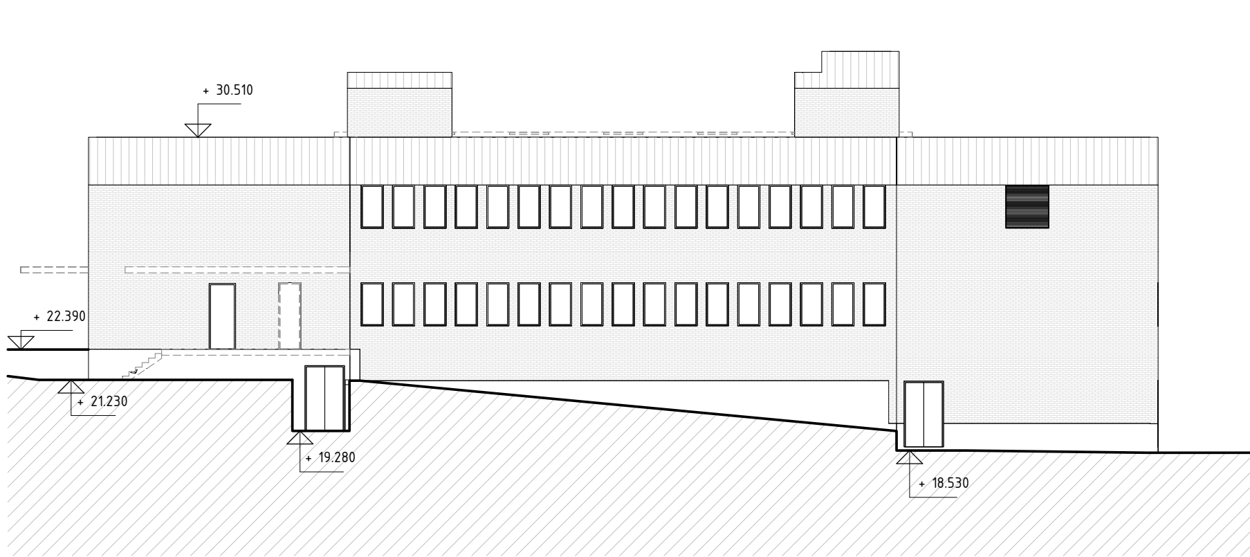
3 - FASAD MOT VÄSTER, BEFINTLIG
