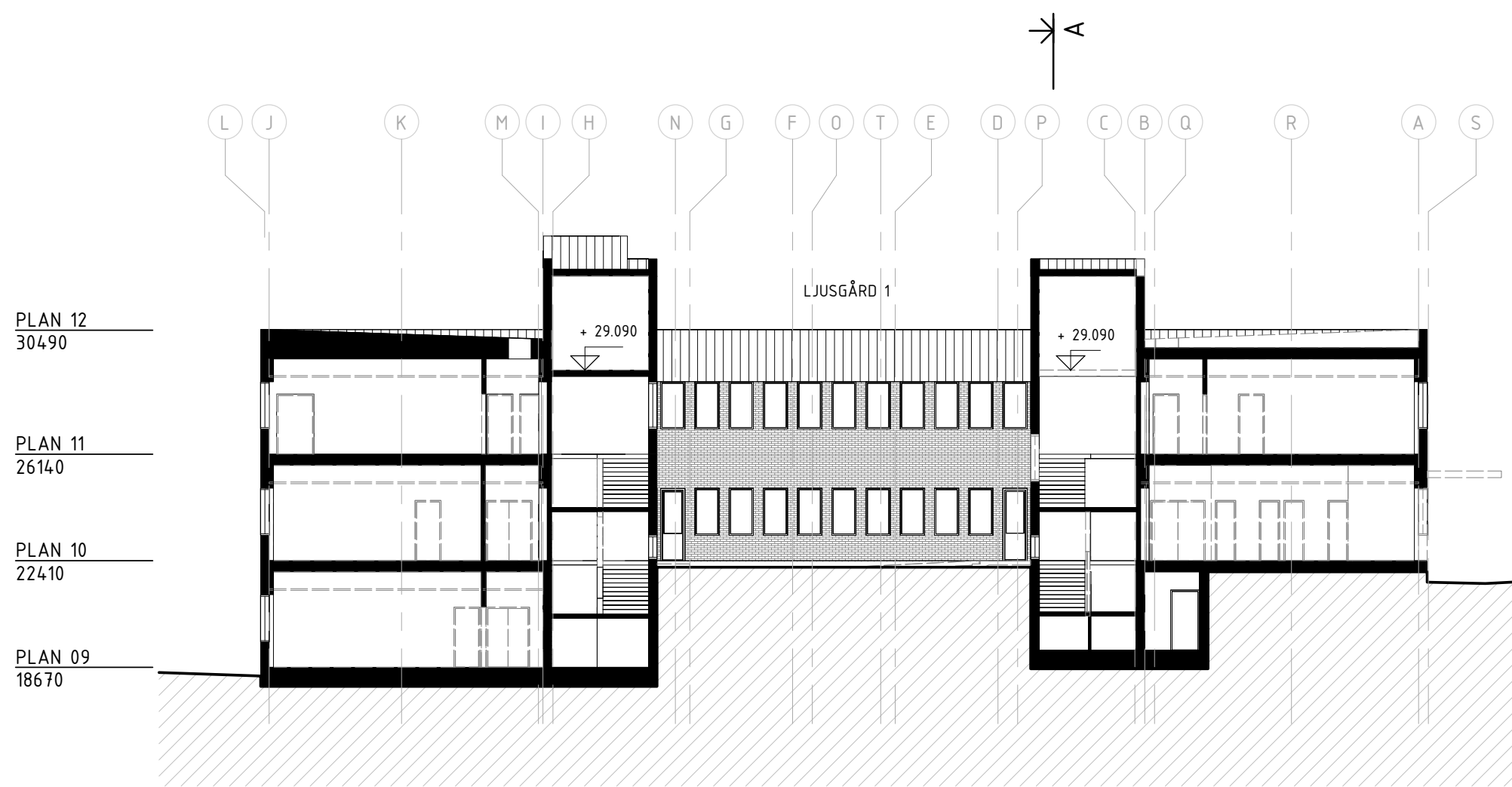
SEKTION B-B, BEFINTLIG
